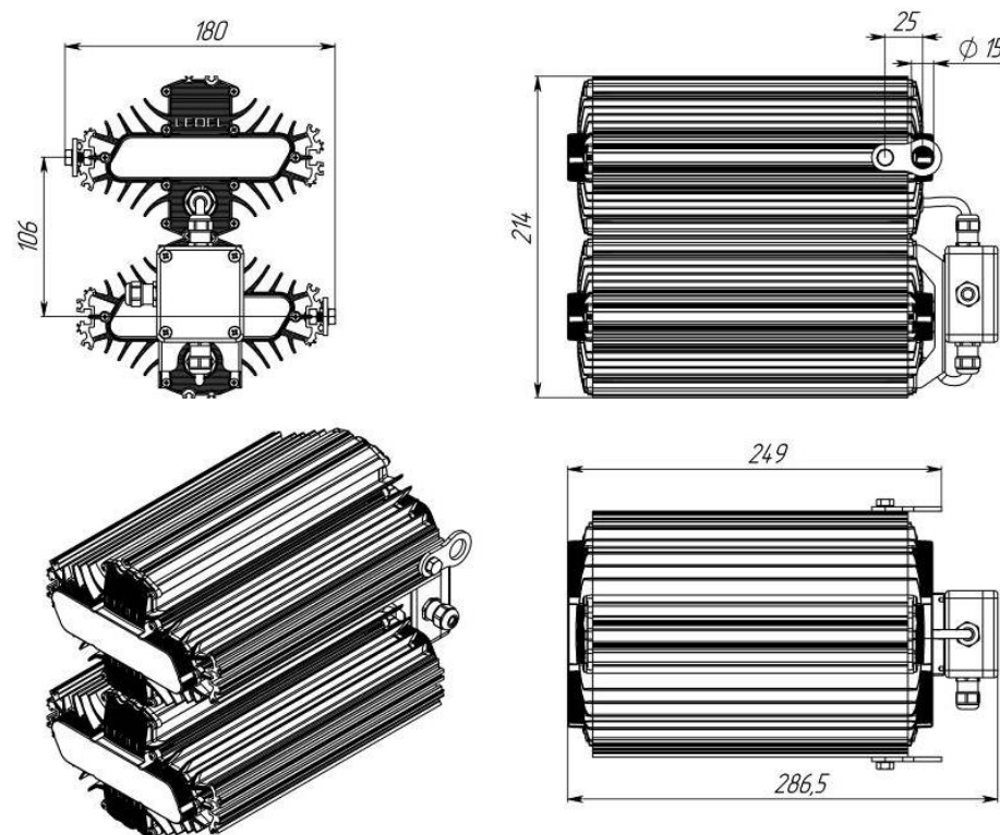
Рисунок. 1 Светильник «L-lego 110» Подвесное крепление
