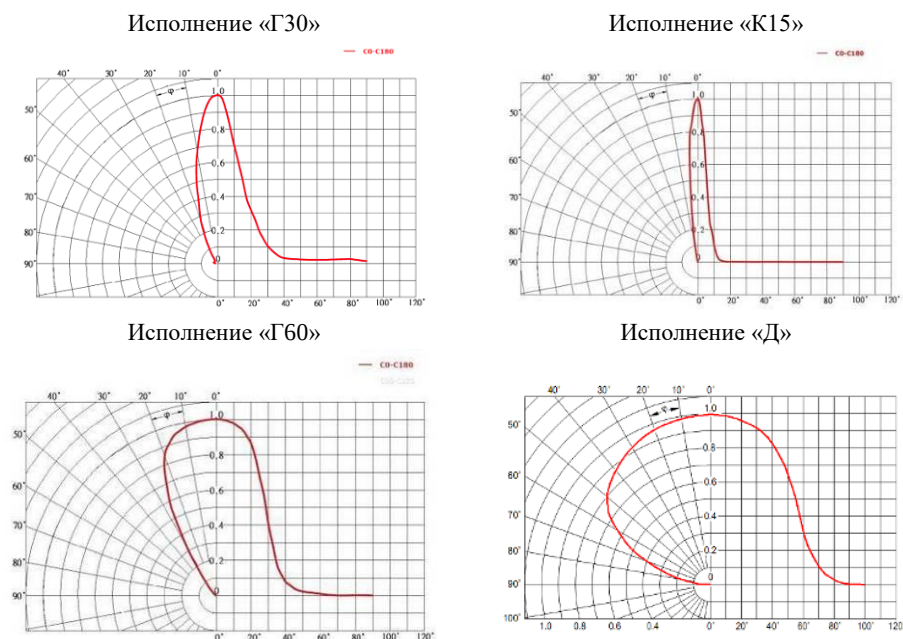
Рисунок 3 Типы КСС
